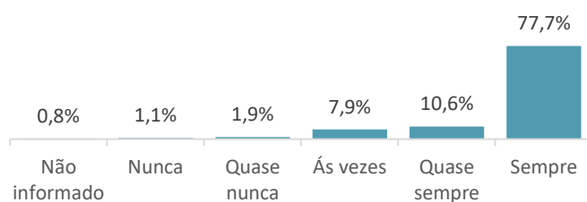
Gráfico 1: Percepção dos adolescentes em relação a sentir acolhidos em casa.
